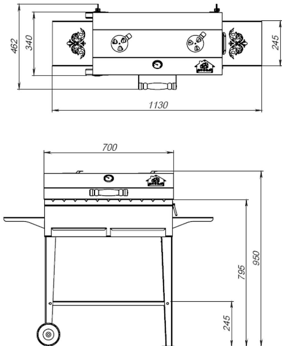
Рис. 1 Габаритные размеры
