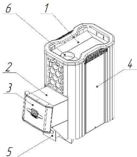
Рисунок 1а - Конструкция печи-каменки «СИБИРЬ (2.0)»
